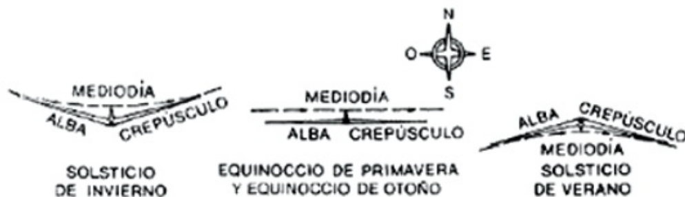
Figura 3. — Movimiento de la sombra del gnomon en las zonas tórridas del hemisferio norte durante las diversas estaciones del año.
