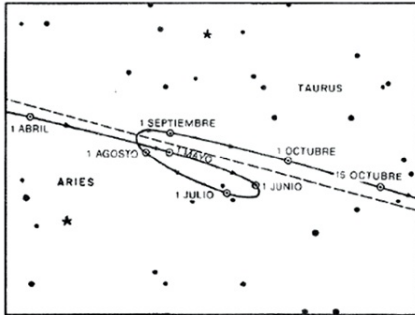
Figura 15. — Retrogradación de Marte a través de las constelaciones de Aries y Taurus. El sector de cielo que aparece en el presente diagrama es el mismo que el de la figura 9 y el encerrado en el recuadro del mapa estelar de la figura 8. La línea de trazo discontinuo es la eclíptica y la de trazo continuo representa la trayectoria del planeta. Obsérvese que Marte no permanece sobre la eclíptica y que, a pesar de que su movimiento general a través de las estrellas se efectúe en dirección este, hay un período, de mediados de junio a comienzos de agosto, en el que se mueve hacia el oeste. Las retrogradaciones de Marte siempre tienen una forma y duración muy similares, pero no siempre se producen en las mismas fechas ni dentro del mismo sector de cielo.
