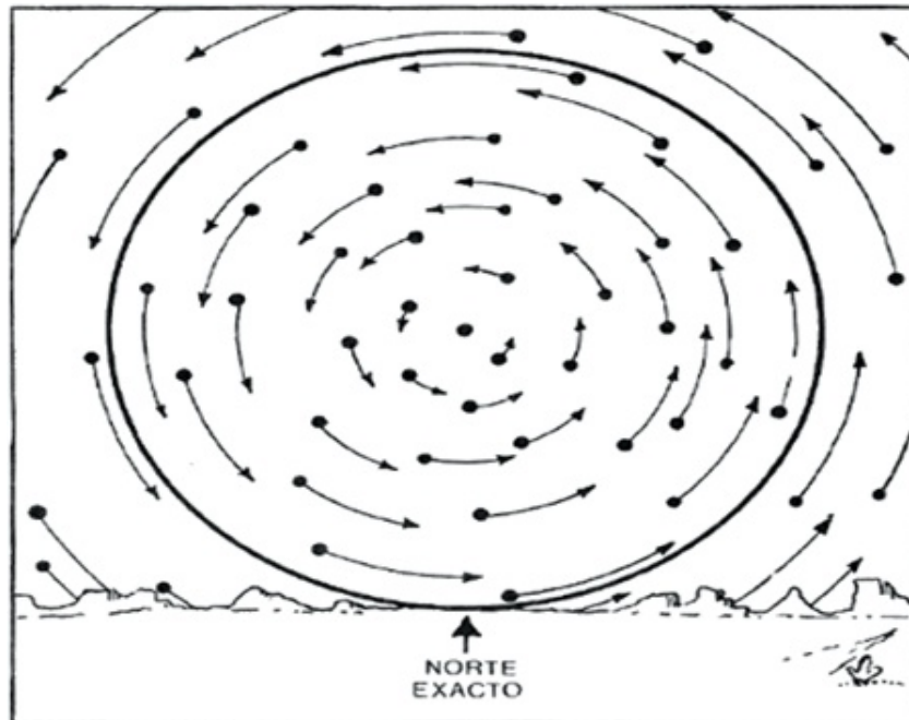
Figura 6. — Conjunto de arcos de círculo descritos por algunas estrellas del hemisferio norte durante un período de dos horas. La circunferencia de trazo grueso tangente al horizonte separa las estrellas circumpolares de las que salen y se ponen. Puede obtenerse una imagen de estas trayectorias estelares mediante una cámara fotográfica con el objetivo dirigido hacia el polo celeste y dejando el obturador abierto mientras gira el conjunto de los cielos. Cada hora suplementaria de exposición alarga en 15^\circ el arco descrito por las estrellas. Sin embargo, debe tenerse en cuenta que la particular orientación del objetivo introduce una engañosa distorsión. Si el polo celeste está situado 45^\circ por encima del horizonte, que es muy aproximadamente el caso en nuestras latitudes, una estrella que en la figura aparece muy cerca de la parte superior del círculo de separación estará en realidad sobre la misma cabeza del observador. Una vez reconocida esta distorsión, que tiene como origen el ángulo dado a la cámara fotográfica, se hace posible relacionar los trazos de trayectoria estelar de este diagrama con los que aparecen de forma más esquemática en las figuras 7a y 7b.
