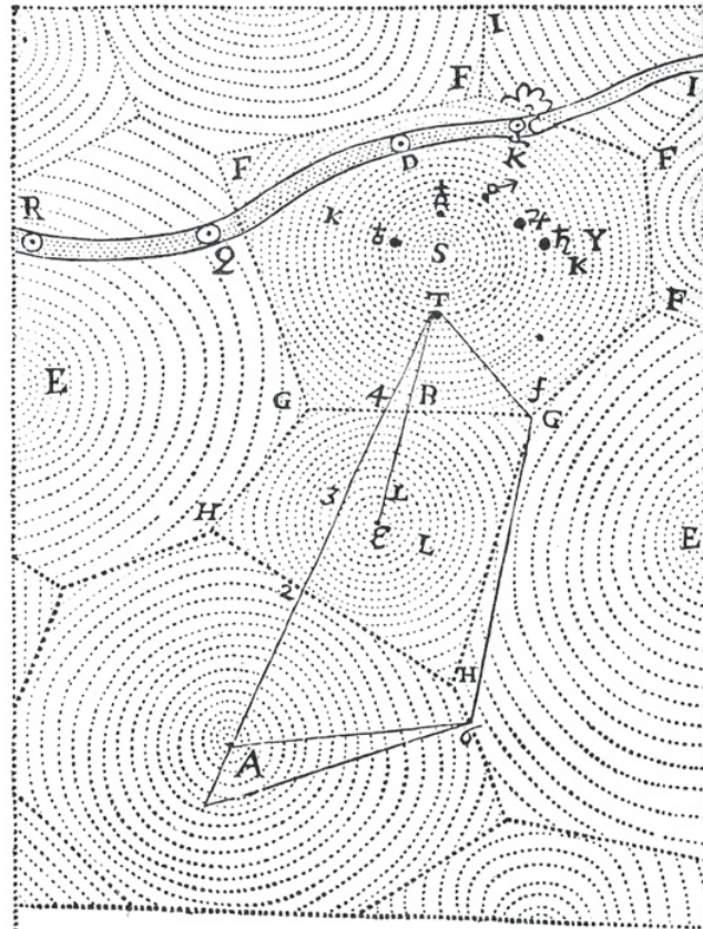
Figura 47. — La cosmología de los torbellinos de Descartes, reproducida de su obra Le monde ou le Traité de la Lumière . Los puntos S, E, A y ε son los centros de los torbellinos. Los rápidos movimientos en torbellino de los corpúsculos centrales los convierten en luminosos, por lo que actúan a modo de estrellas. Los diversos círculos punteados, que no es necesario que conformen circunferencias perfectas, representan los caminos descritos por las corrientes corpusculares, eternamente en rotación, que constituyen el torbellino. Los puntos negros situados alrededor del centro S del torbellino son los planetas, que se ven arrastrados a lo largo de sus respectivas órbitas por el movimiento de los torbellinos. El cuerpo C, situado en la parte superior del diagrama, es un cometa que atraviesa los diferentes torbellinos en una región en la que su movimiento es demasiado lento para constreñirlo sobre una órbita circular continua. El espacio exterior al diagrama está asimismo lleno de torbellinos y cada uno de ellos, al menos potencialmente, representa la localización de un sistema solar en el seno del universo copernicano de Descartes poblado por una infinidad de mundos.
