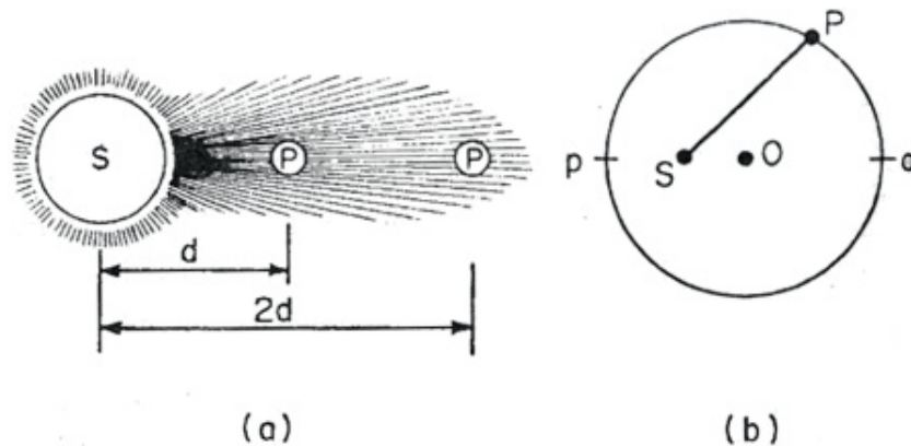
Figura 41. — La primitiva ley de velocidades enunciada por Kepler. El diagrama (a) muestra los rayos del anima motrix que emanan del sol, ilustrando la teoría física de la cual Kepler dedujo su ley. El diagrama (b) muestra en qué forma puede ser aplicada esta ley a un planeta que se mueva sobre una excéntrica.
