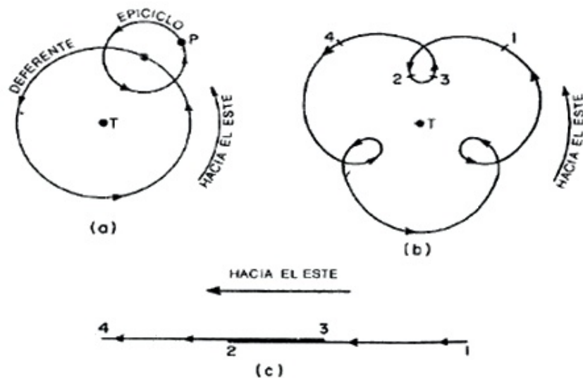
Figura 19. — El sistema básico epiciclo-deferente. En (a) se representa un caso típico de epiciclo y deferente; en (b) aparece el movimiento en bucle generado por tal sistema en el plano de la eclíptica; en (c), se ofrece parte del movimiento representado en (b), el trayecto 1-2-3-4 tal como es visto por un observador situado sobre la tierra central T.
