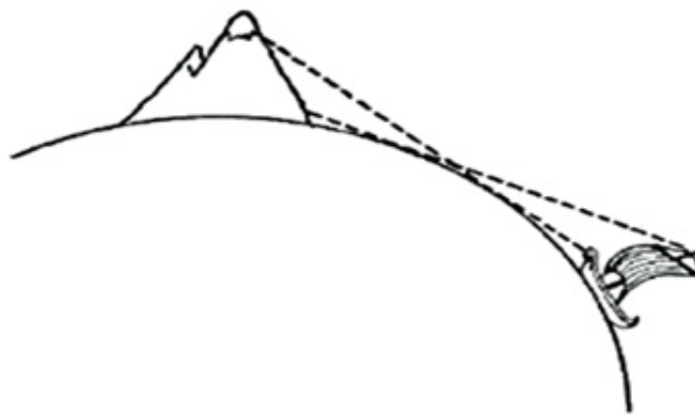
Figura 10. — Antigua prueba (y también moderna) en favor de la esfericidad de la tierra. Un observador situado al pie de la montaña sólo puede ver la parte superior del mástil por encima de su horizonte, mientras que si se halla en la cima del monte se le hacen visibles todo el mástil y parte del casco.
