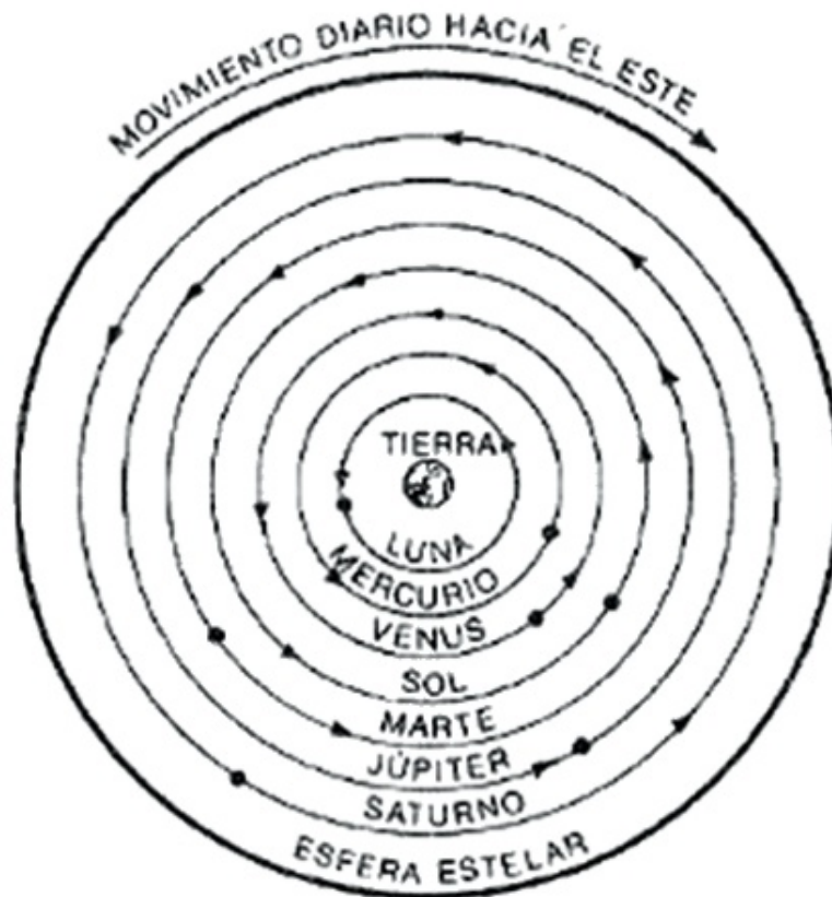
Figura 16. — Esquema aproximado de las órbitas planetarias en el universo de las dos esferas. El círculo exterior es una sección recta de la esfera de las estrellas en el plano de la eclíptica.
