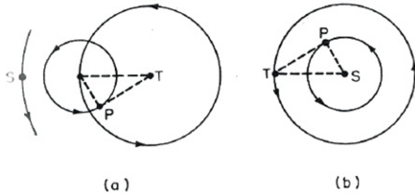
Figura 35. — Explicación de la elongación límite de los planetas inferiores en el sistema de Ptolomeo (a) y en el sistema de Copérnico (b.) En el sistema ptolomeico es necesario limitar arbitrariamente el ángulo entre el sol S y el planeta P manteniendo el centro del epiciclo sobre la recta que une la tierra con el sol. En el sistema copernicano no es necesario imponer tal restricción porque la órbita del planeta se halla contenida por completo en la de la tierra.
